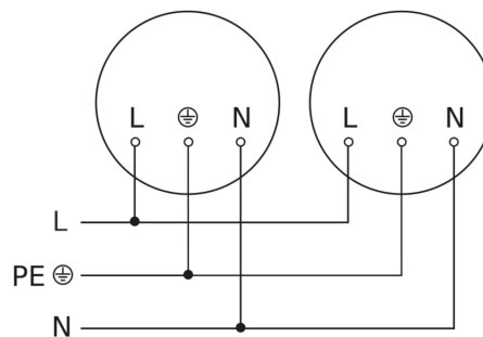
Schema elettrico Master-Slave collegamento in rete
